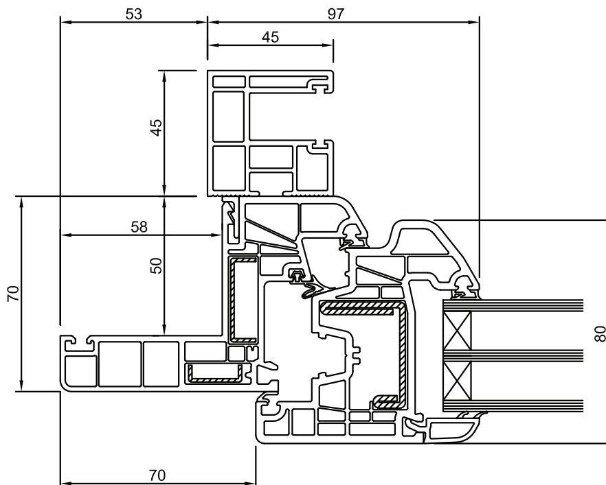
TELAIO Z 58 CON GUIDA AVVOLGIBILE IN PVC
