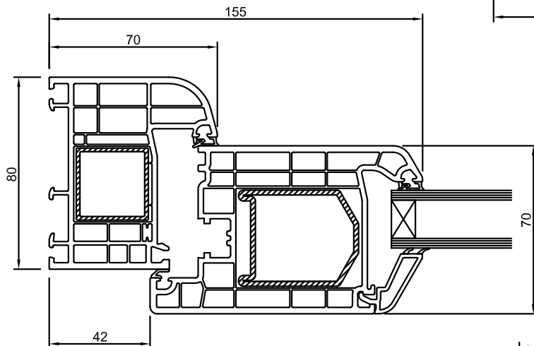
VENERE PLUS TELAIO PIANO CON ANTA MAGGIORATA (PORTONCINO)
