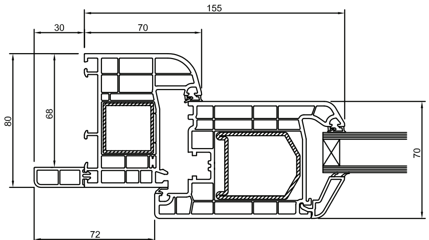
VENERE PLUS TELAIO Z 30 CON ANTA MAGGIORATA (PORTONCINO)
