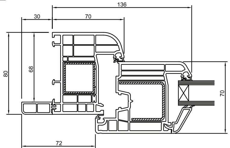
VENERE PLUS TELAIO Z 30 CON ANTA INTERMEDIA (PORTABALCONE)
