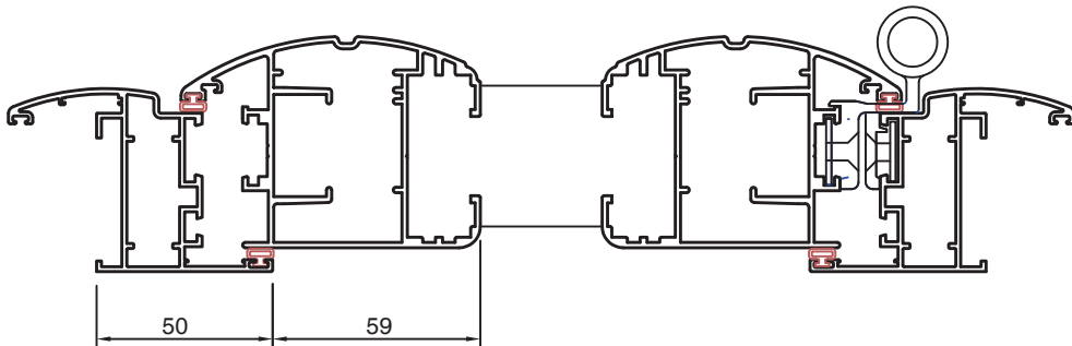
SEZIONE ORIZZONTALE PERSIANA 1 ANTA
