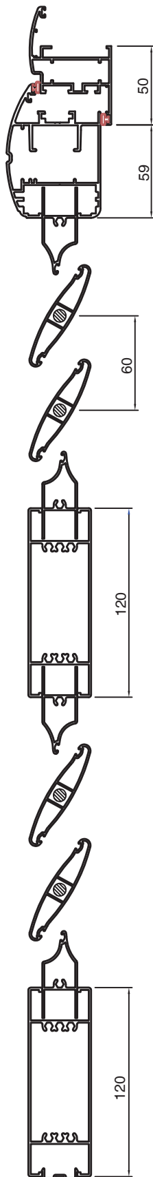
SEZIONE VERTICALE PORTA
