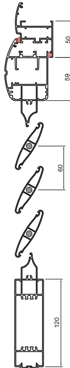
SEZIONE VERTICALE FINESTRA
