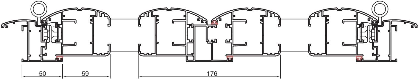
SEZIONE ORIZZONTALE PERSIANA 2 ANTE
